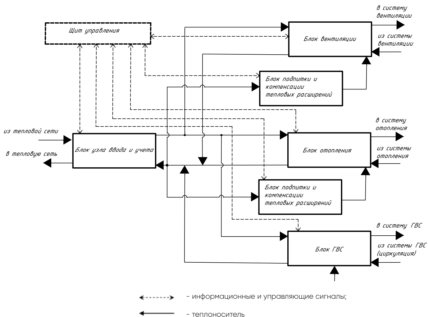
Рисунок 2. Обобщенная структурная схема БТП
